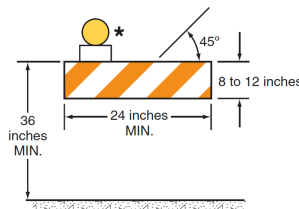
TYPE 1 BARRICADE **
