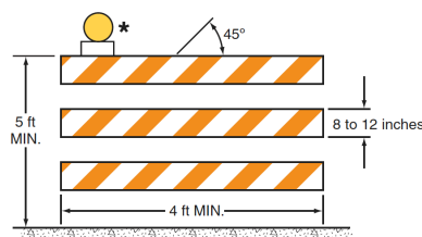
TYPE 3 BARRICADE **
