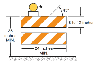
TYPE 2 BARRICADE **
